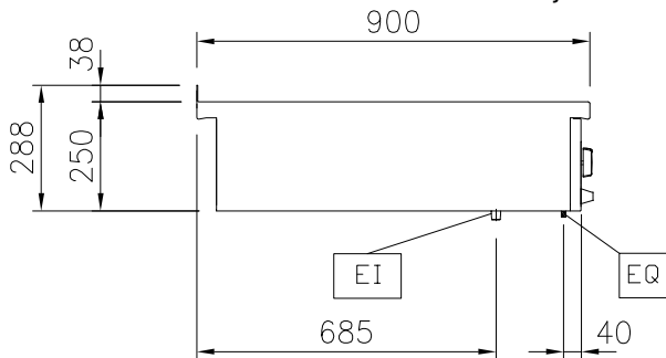
Zij aanzicht
